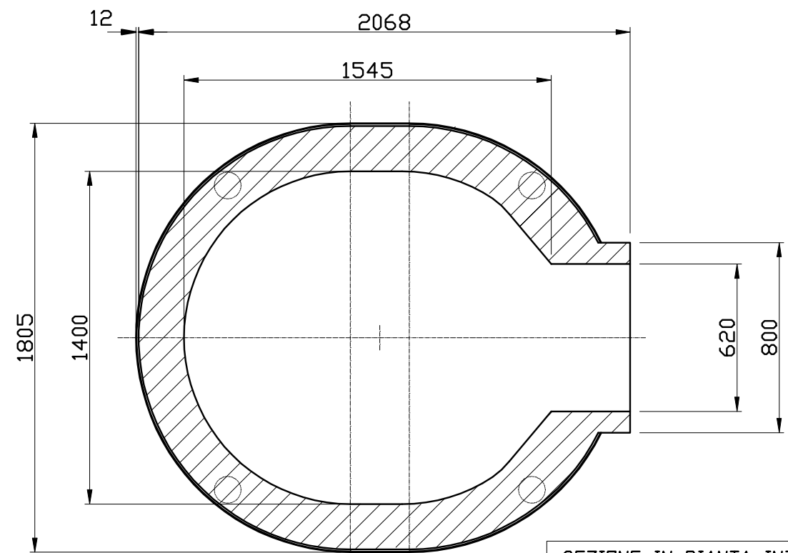
SEZIONE IN PIANTA INTERNO FORNO
